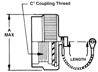
TF261 RECEPTACLE CAP
